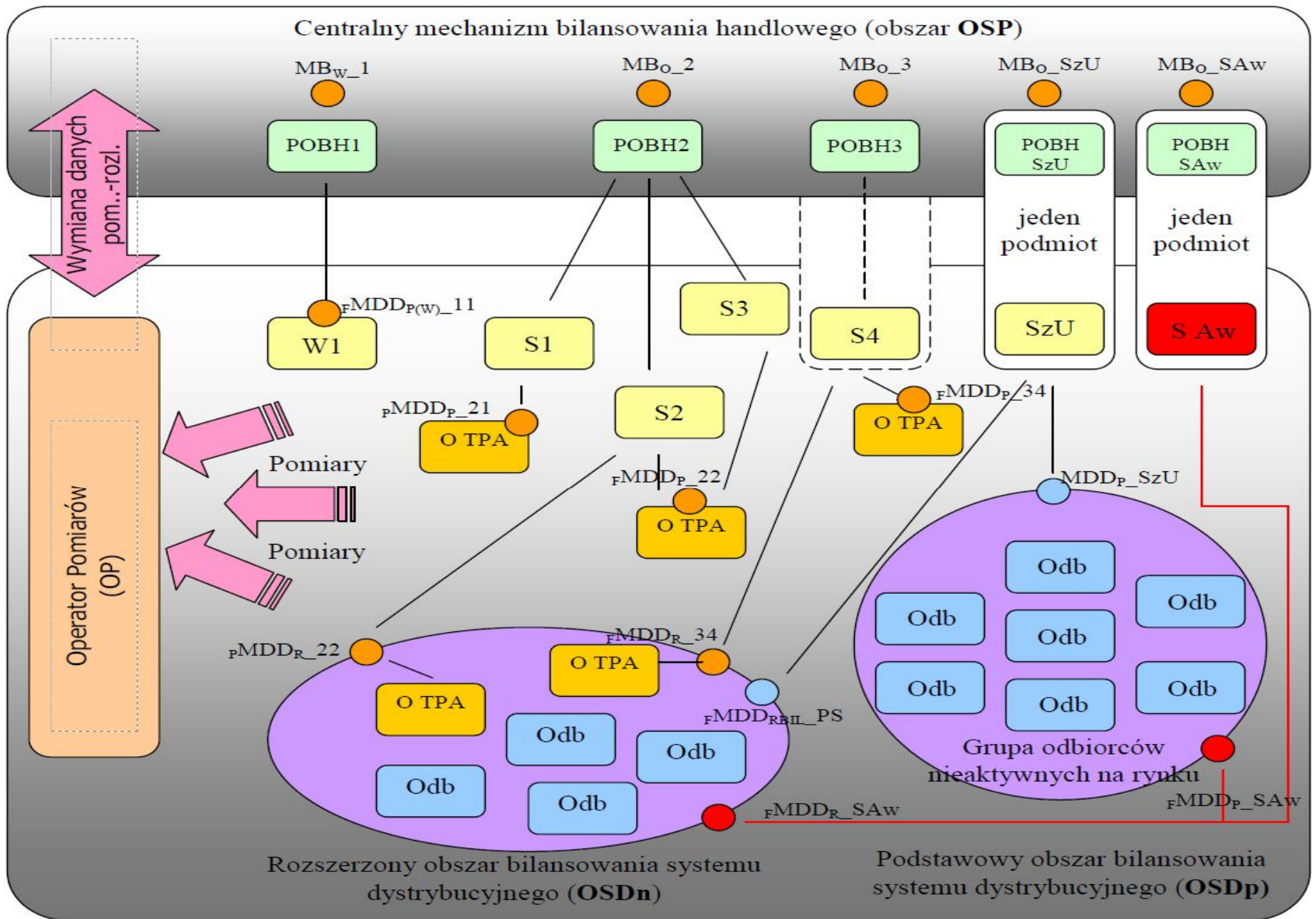
Rys. 2. Uproszczony schemat funkcjonalny współpracy pomiędzy OSP, OSDp i OSDn w zakresie przekazywania danych pomiarowych odbiorców końcowych i wytwórców z podstawowego i rozszerzonego obszaru bilansowania w systemie dystrybucyjnym
